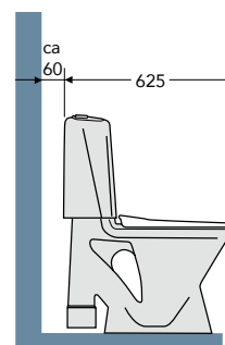
GOLVMONTERAD STANDARD TOALET
